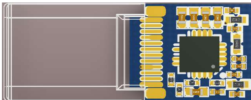
TOP视图
