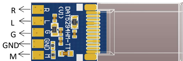
bottom视图
